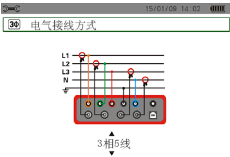
图 5-6 电气连接方式选择
