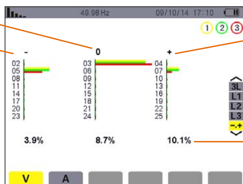
图 7-10 相电压的专家模式显示
