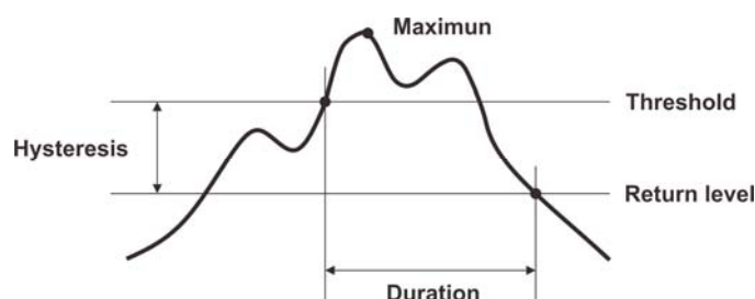
图 17-1 骤升侦测回差图例
