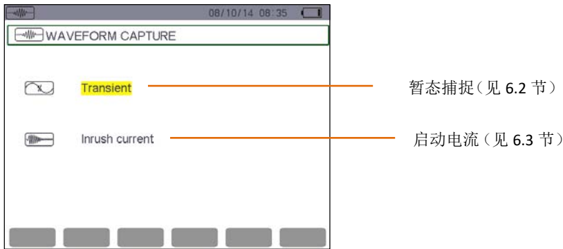
图 6-1 波形捕捉模式
