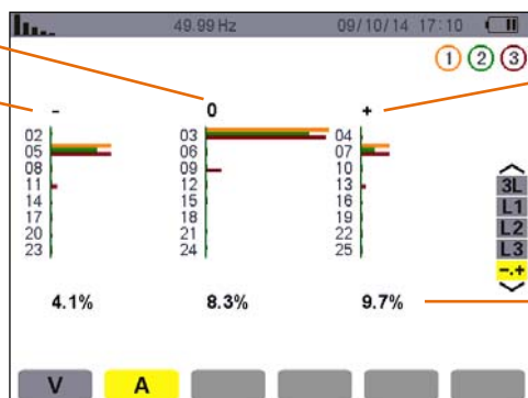
图 7-11 电流的专家模式显示
