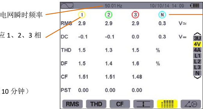
图 8-17 4V 下各值同时显示屏幕
