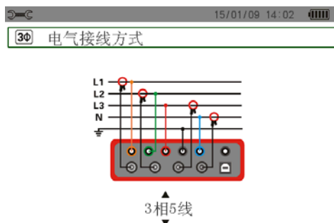
图 4-7 三相5线连接
