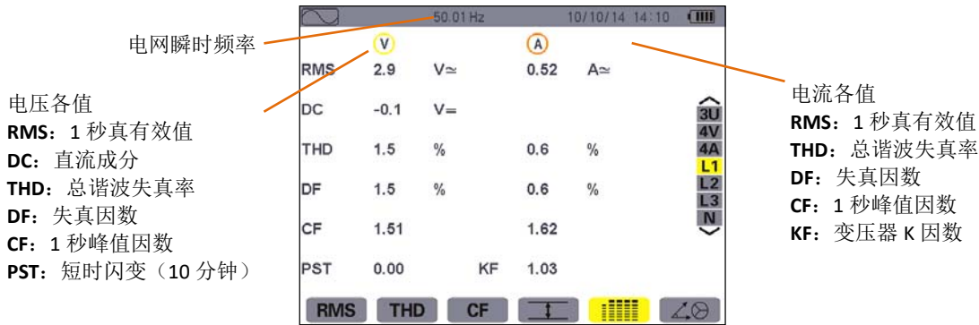
图 8-19 L1 下各值同时显示屏幕
