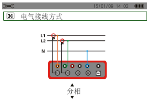
图 4-5 分相连接
