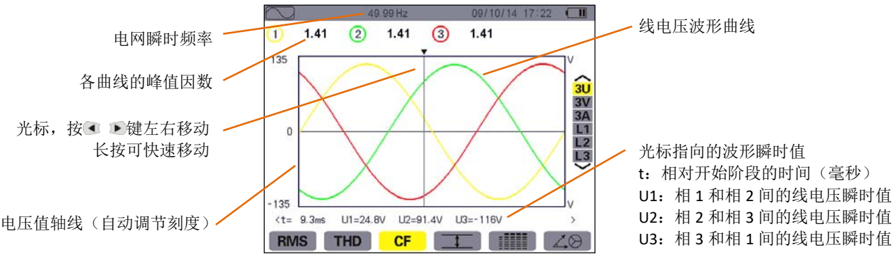
图 8-9 3U 下 CF 显示屏幕
