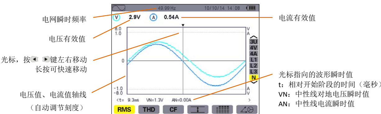
图 8-5 RMS 显示中性线屏幕
