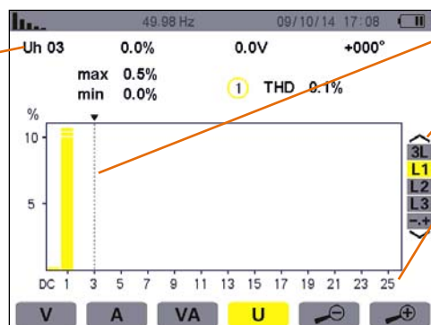
图 7-9 线电压谐波 L1 显示
