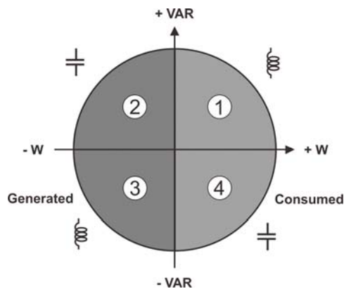
图 17-3 功率电能象限图
