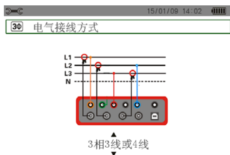
图 4-6-2 三相3线
