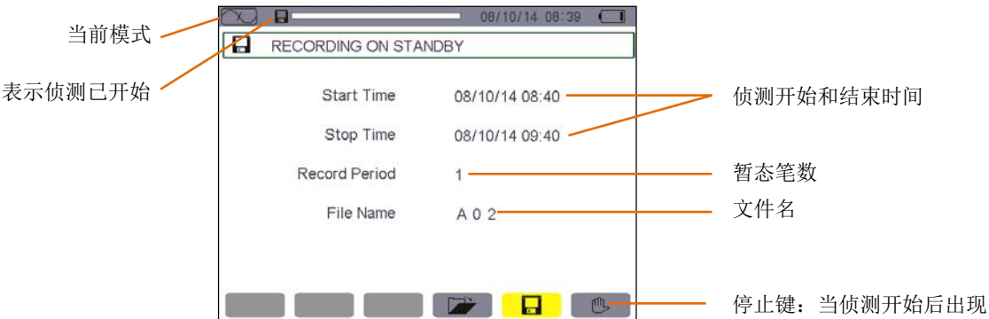
图 6-3 暂态排程进行中
