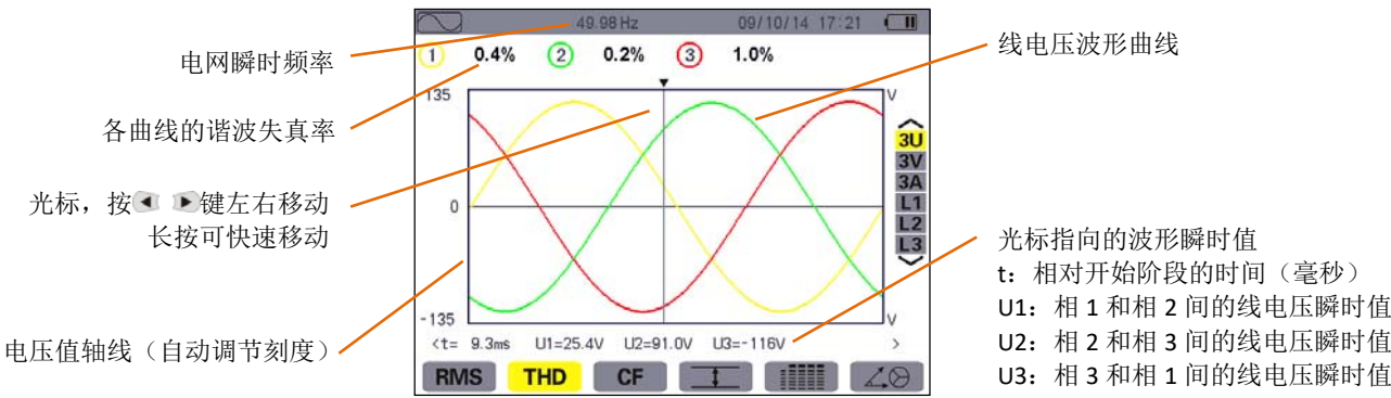
图 8-6 3U 下 THD 显示屏幕
