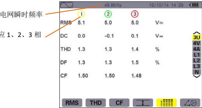
图 8-16 3U 下各值同时显示屏幕
