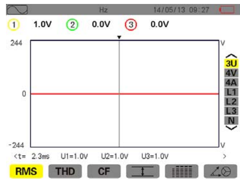
图 4-1 波形图屏幕
