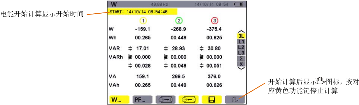
图 11-9 开始电能计算时的功率和电能显示屏幕
