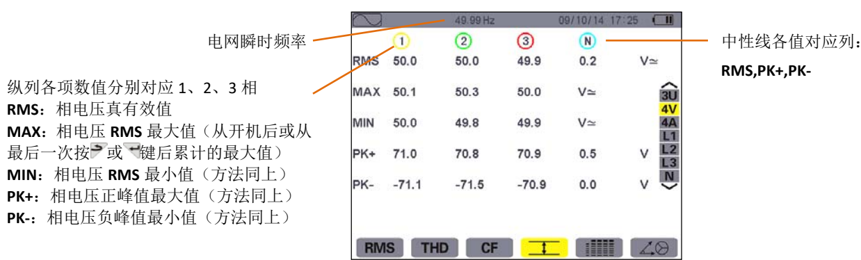
图 8-13 4V 下 Max.-Min.显示屏幕
