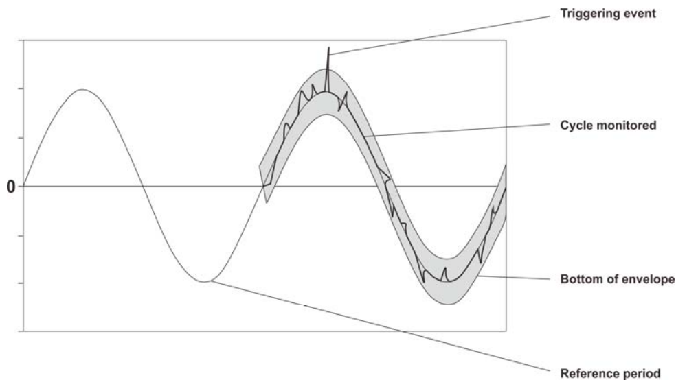
图 17-4 暂态捕捉触发原理图解
