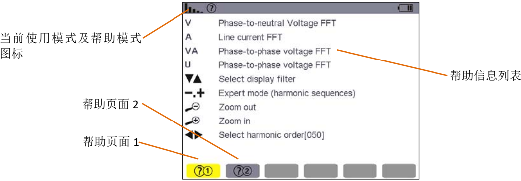
图 13-1 谐波模式下帮助页面图例，第一页
