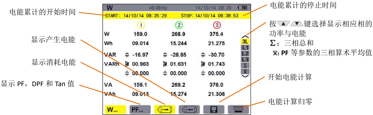
图 11-1 功率和电能屏幕
