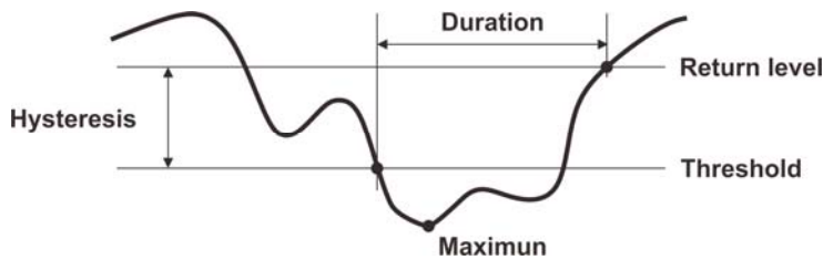
图 17-2 骤降侦测回差图例
