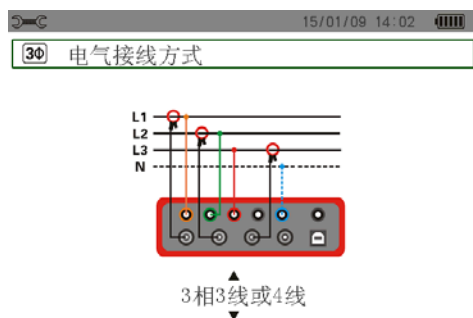
图 4-6-1 三相4线
