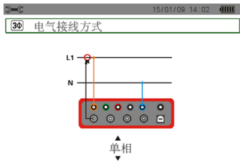
图 4-4 单相连接
